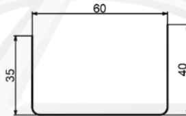
Biên dạng U 60-40-35 - khổ 130
